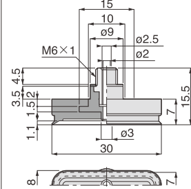
VP 8×30E□A
