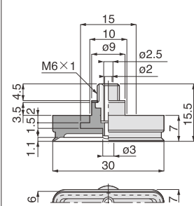
VP 6×30E□A
